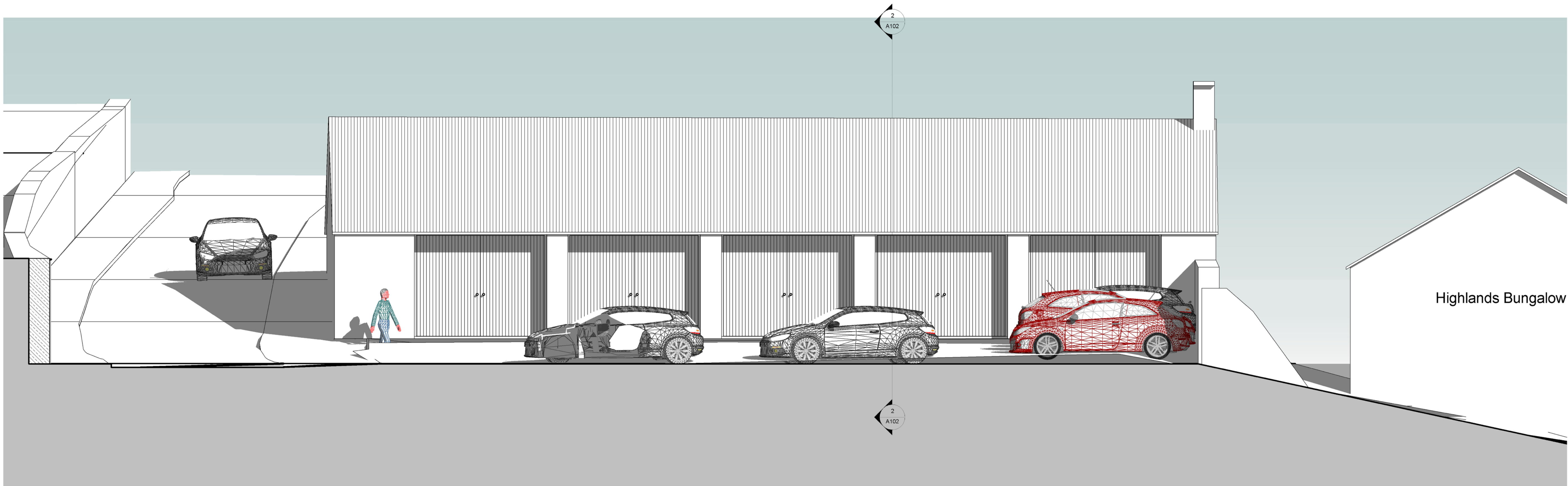
1 Section 1 1 : 50
