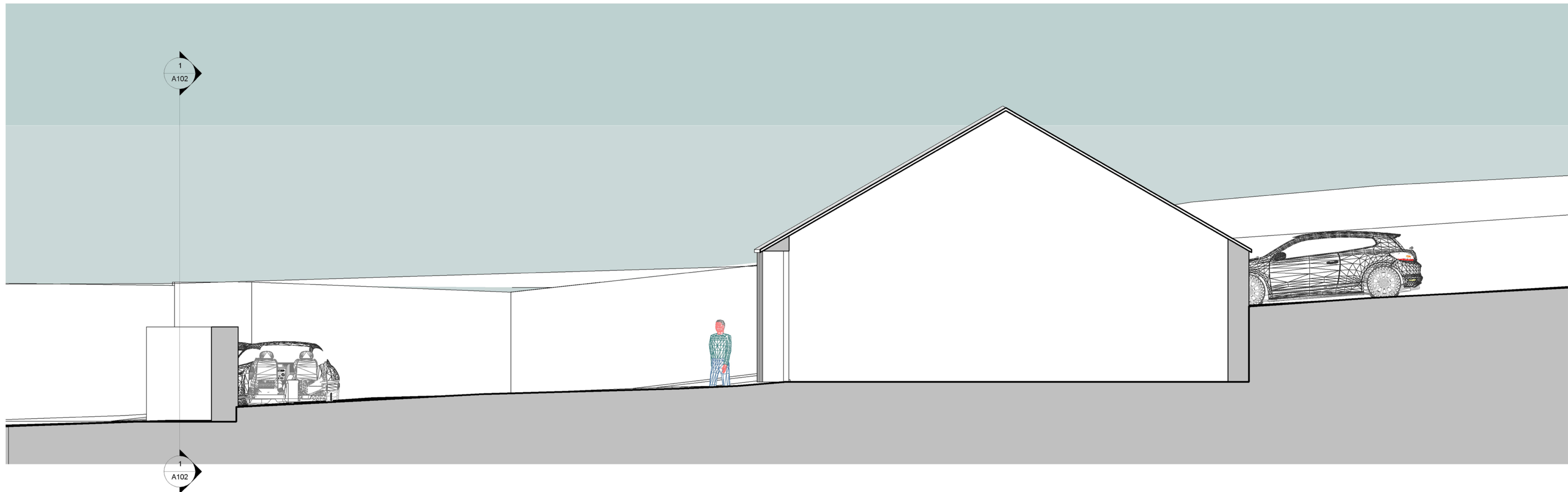
2 Section 2 1 : 50
